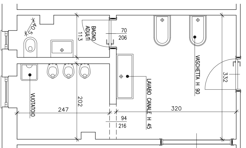
SC 1:150 DETTAGLIO BLOCCO BAGNO 3
